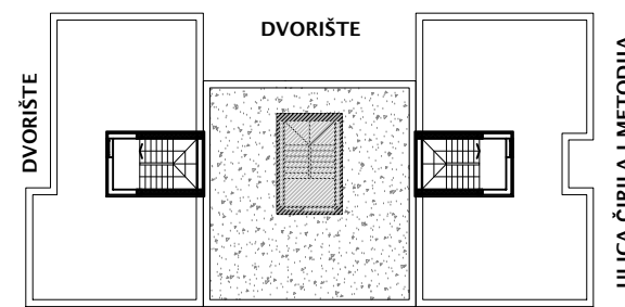
OSNOVA DUPEKSA
