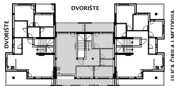
OSNOVA POTKROVLJA
