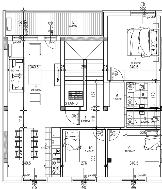
OSNOVA POTKROVLJA
