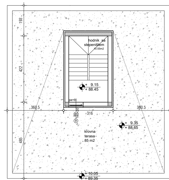
OSNOVA DUPEKSA
